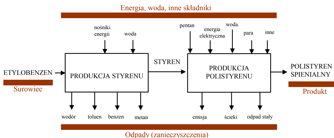
Rys. 2. Etapy procesu produkcyjnego
